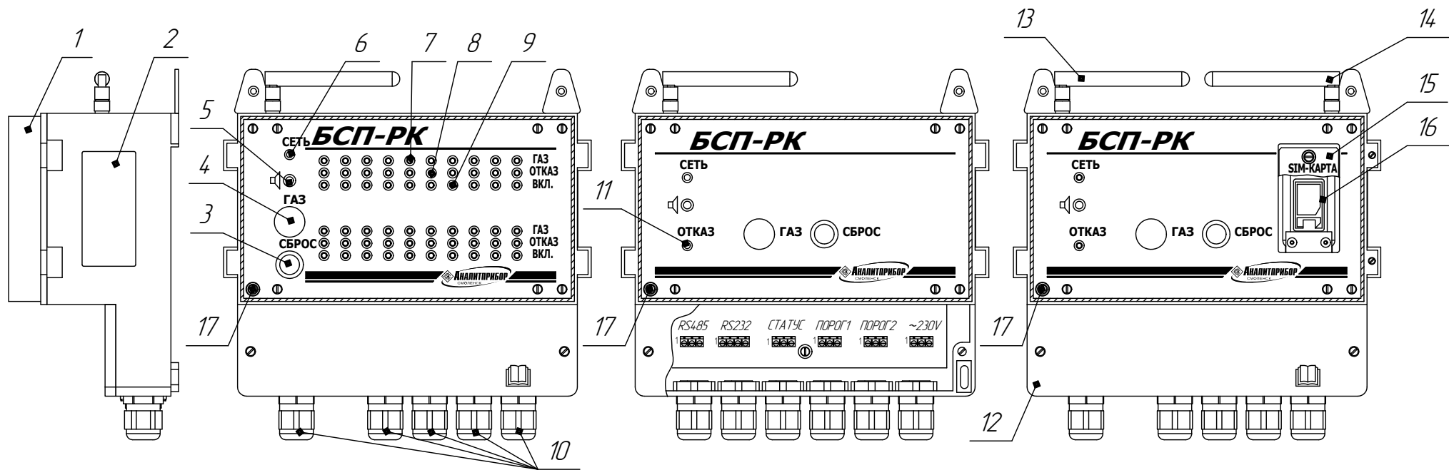
в) блок БСП-РК-03
